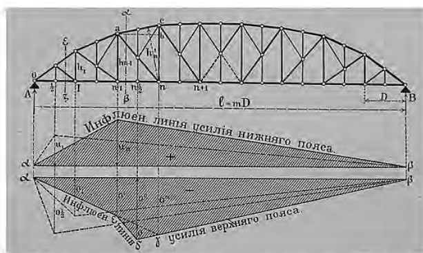
Il. 7. Plany budowy mostu na Jenisieju – fragment.
