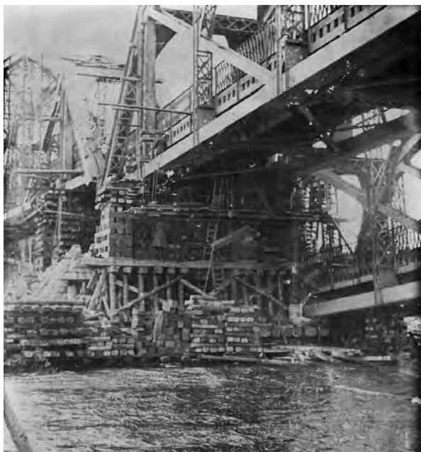
Il. 16. Prace remontowe przy moście na Bugu. Źródło: Zbiory Artura Soszyńskiego.
